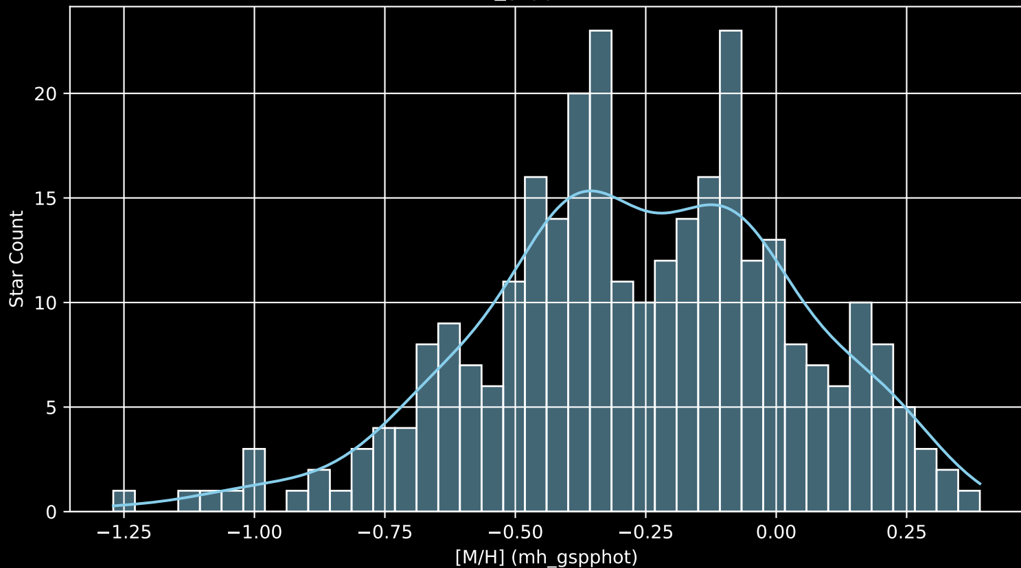
GALAH DR4 Field: [212] [M/H] (mh_gspphot) (n= 297)
