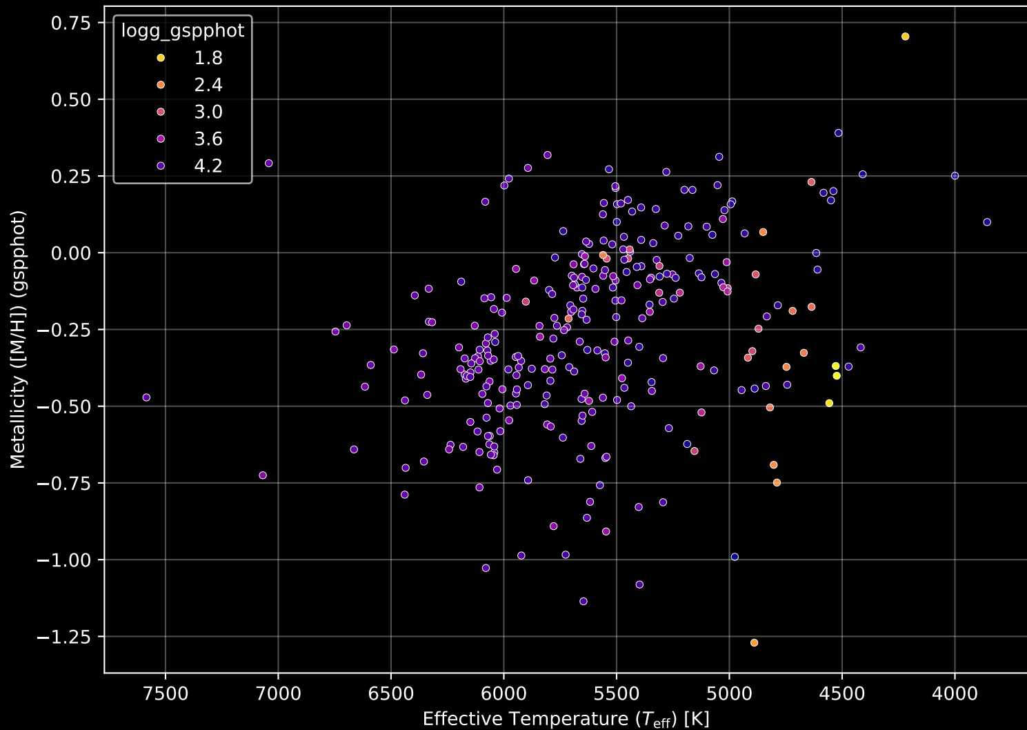
GALAH DR4 Field: [212] Stellar Population Parameters (n= 298)
