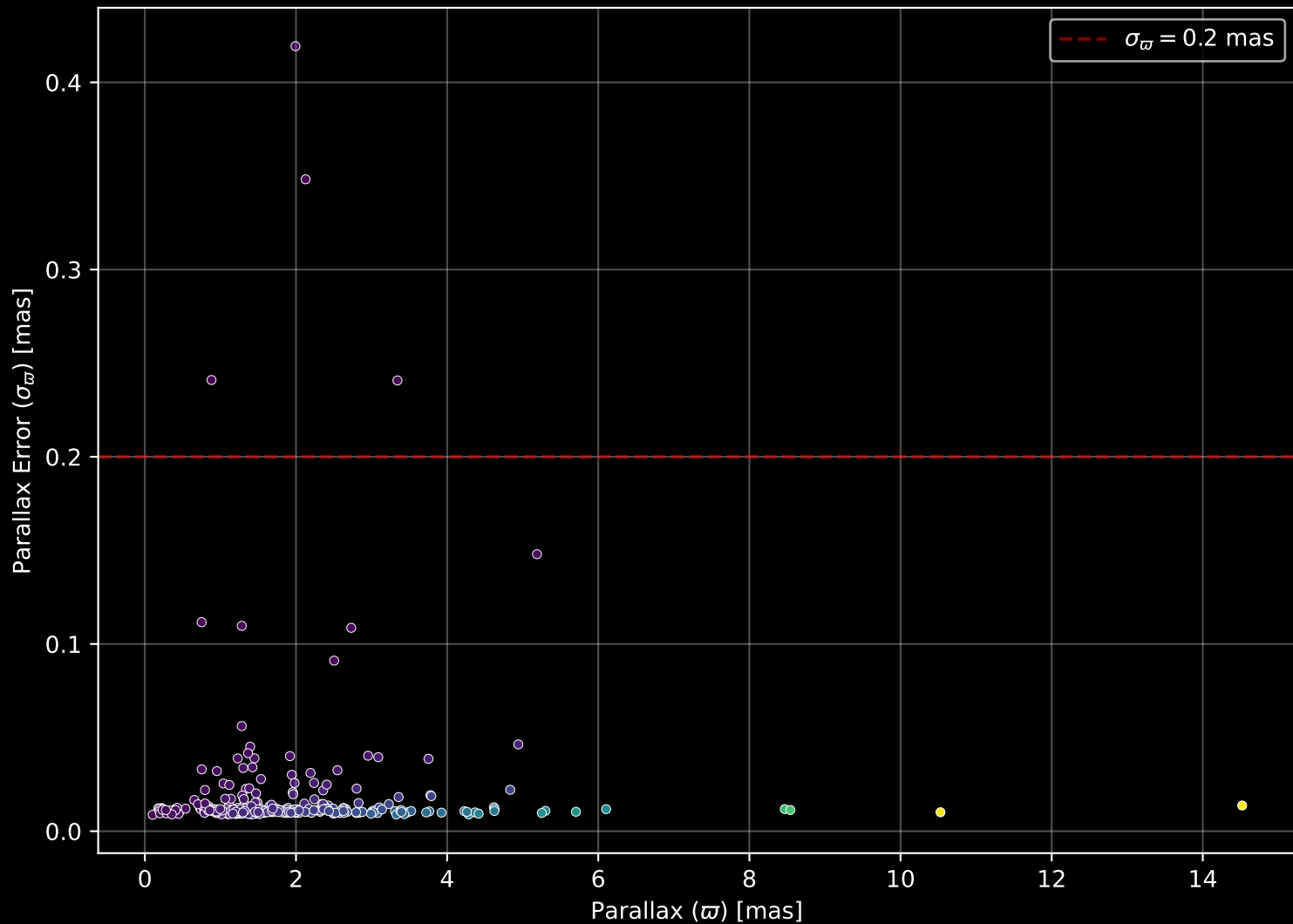
GALAH DR4 Field: [212] Parallax Quality (n= 298)
