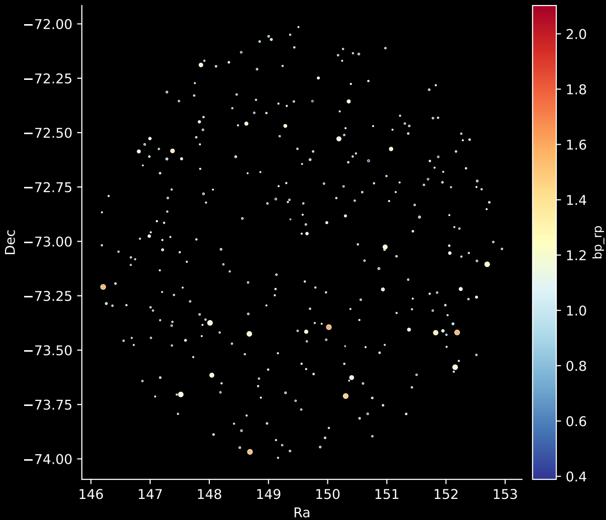
GALAH DR4 Field: [212] Stars: 298
